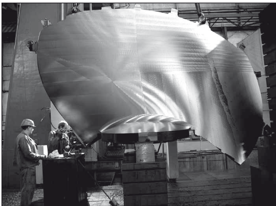
Hrubovaný odliatok lopatky Kaplanovej turbíny.
