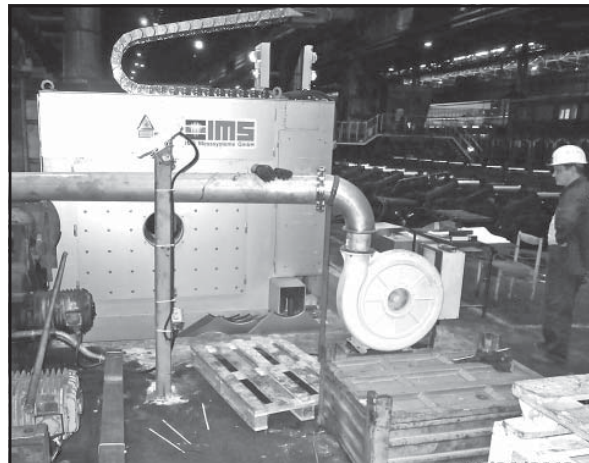
Pohľad na montáž nového IMS - č.1 pred pecou redukovne. Nové zariadenie na meranie hrúbky steny lupy pred redukovňou. Foto: J. Búlik
