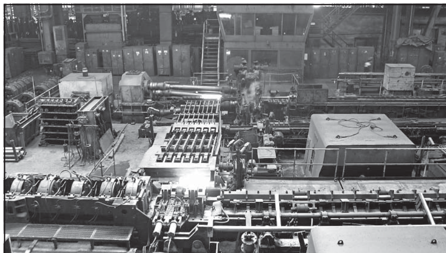
Pohľad do valcovne bezšvíkových rúr objektívom A. Nociarovej
