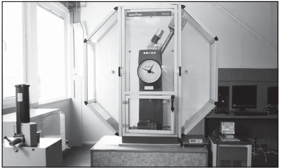
Zariadenie na skúšky vrubovej húževnatosti ocele.
