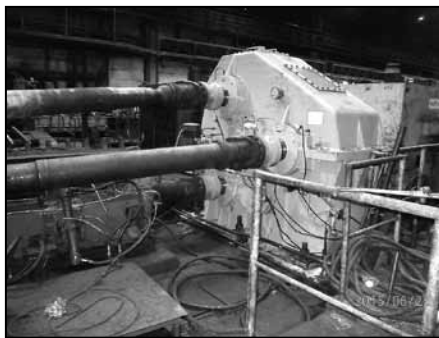
Vymenená prevodovka pohonu valcov elongátora vo valcovni rúr objektívom J. Romančíka
