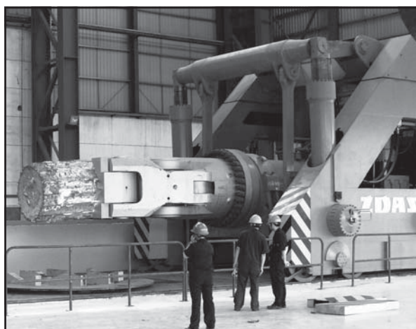
Manipulátor QKK 100 vo firme WHHI Wuhan je meradlom súčasných možností výrobného potenciálu firmy ŽDAS, a.s.
