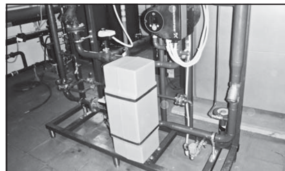
Novoinstalovaná výmenníková stanica tepla v budove energetiky využívajúca odpadové teplo z odprášená. Foto: archív Te
