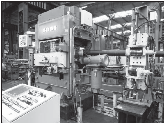
Montáž rovnačky XRK 2 - 90 pre čínskeho zákazníka. Foto: J. Šindelka
