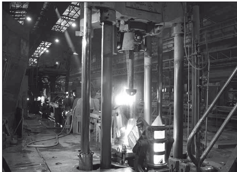
Od 8. marca vo valcovni bezšvíkových rúr pracujú opäť v nepretržitom štvorčatovom pracovnom režime Ilustračné foto: A. Nociarová
