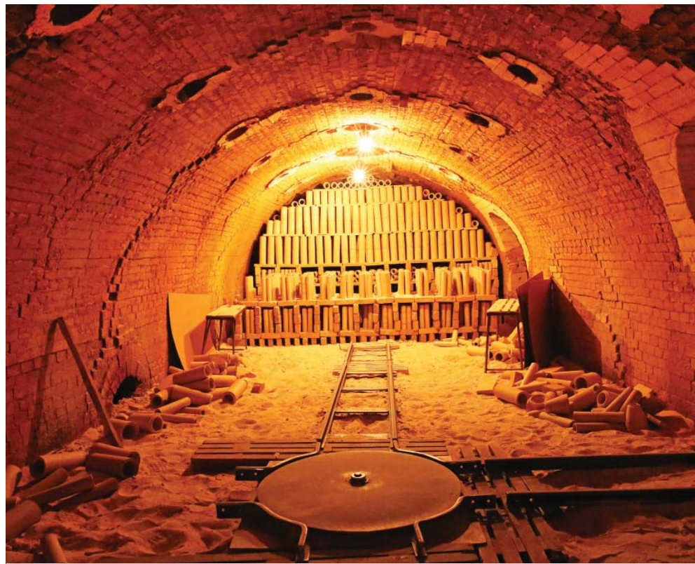
Kruhovú pec na vypaľovanie šamotu
